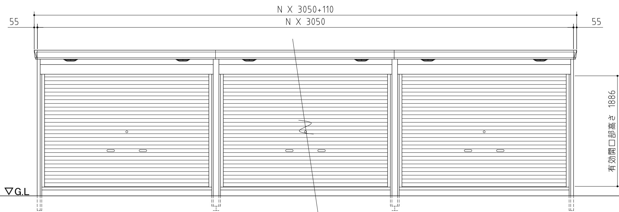
正面図
