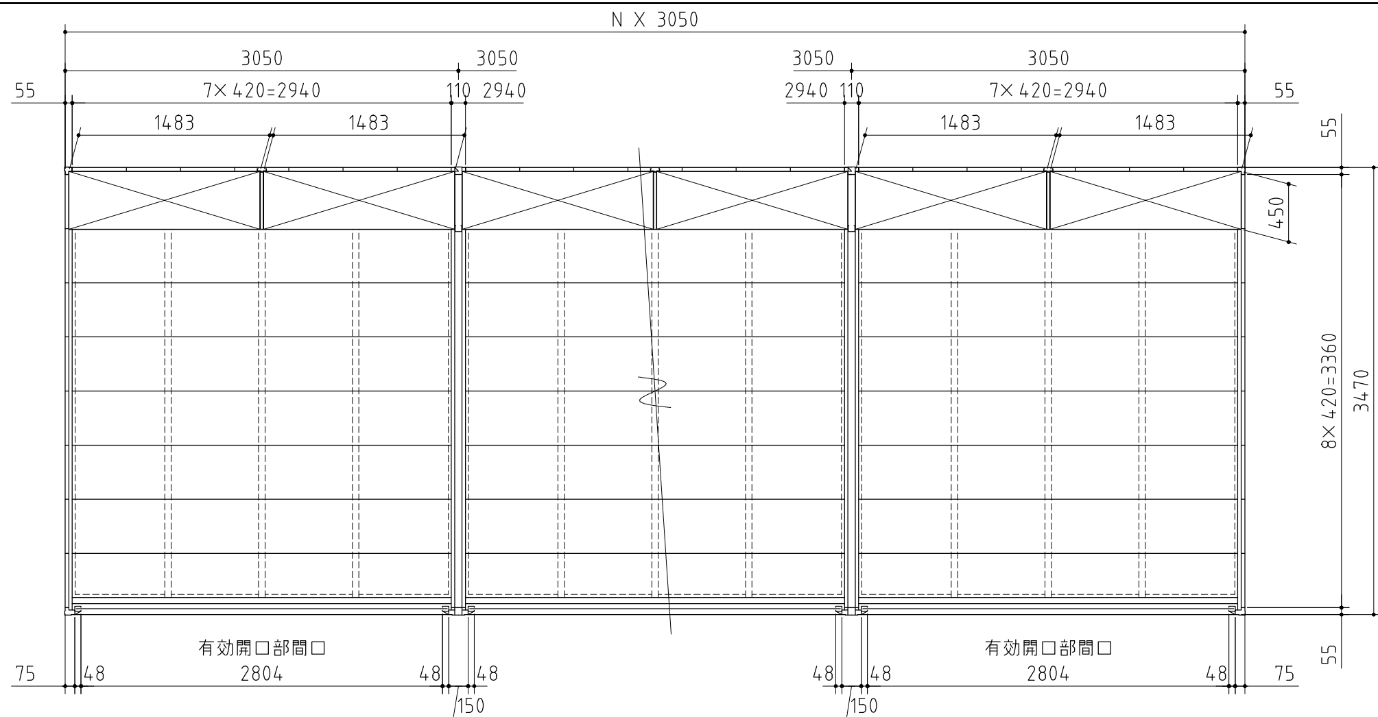
平面図
